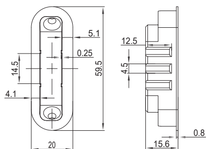
Ответная планка
